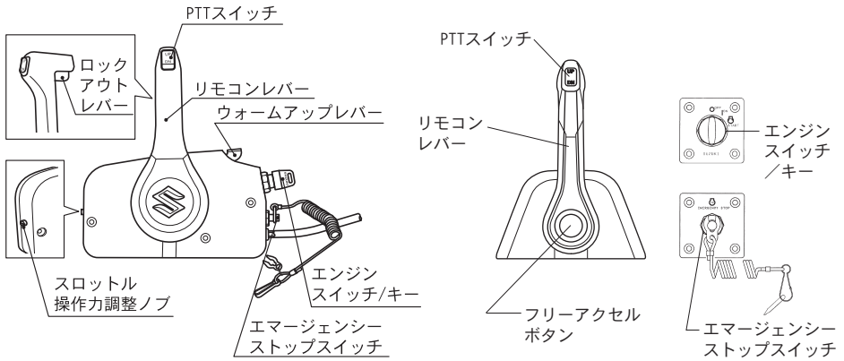
サイドマウントタイプ リモートコントロールボックス仕様
