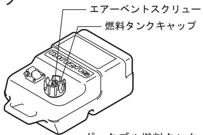
ポータブル燃料タンク
