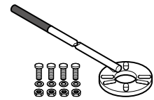
09930-48720 フライホイールホルダー Applicable Model DF25A-90A
