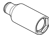
09922-21410 ロングソケットレンチ Applicable Model DF350A
